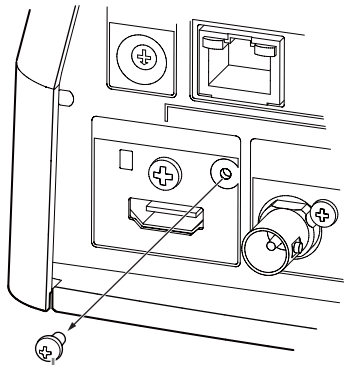
HDMI 电缆锁定螺钉（M2.6 × 6、黑色）
